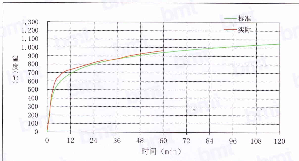
图1 炉内升温曲线
