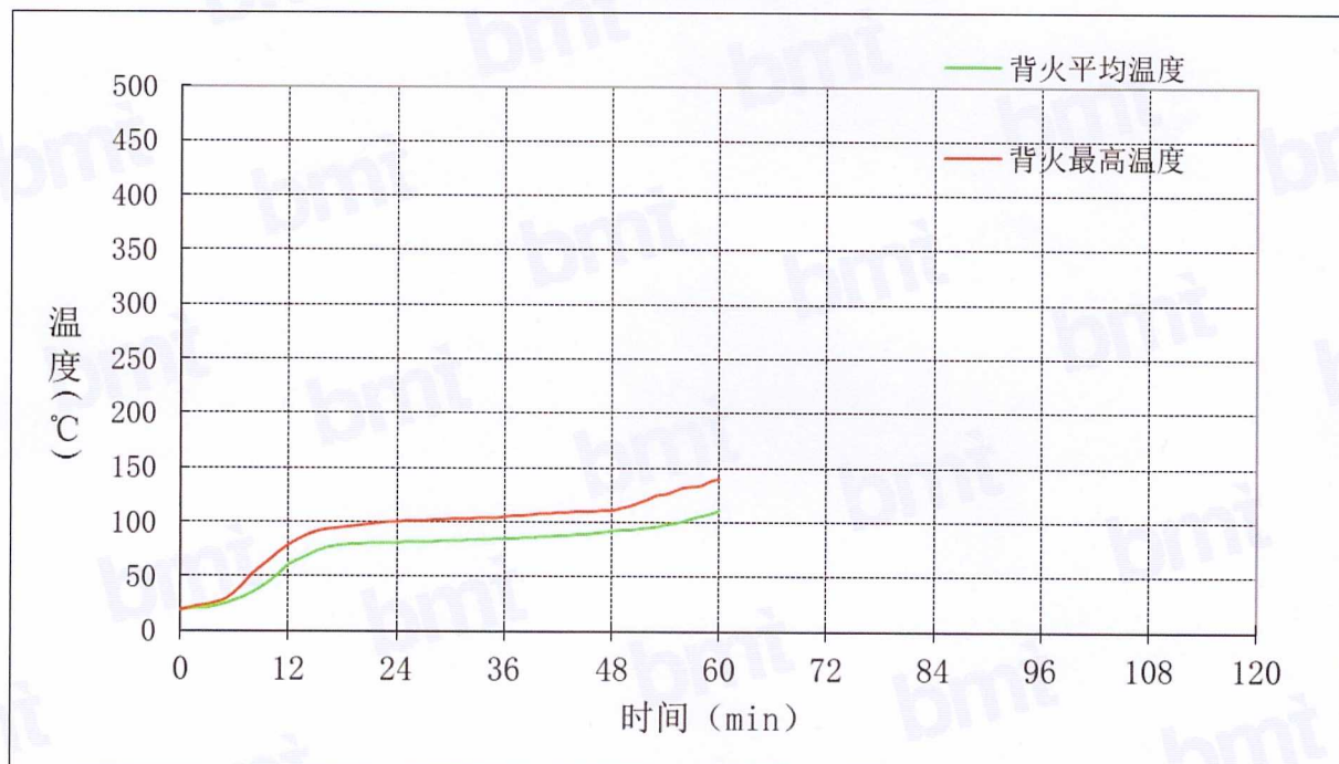
图2 背火温升曲线
